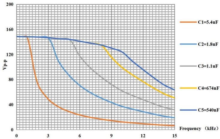
ATA-P1005 容性负载曲线图
