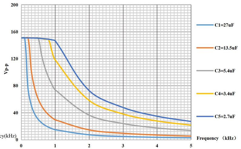
ATA-P0102 容性负载曲线图
