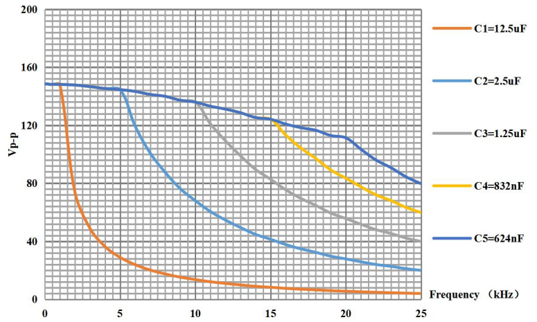
ATA-P2010 容性负载曲线图
