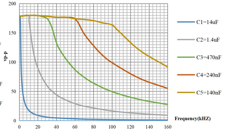
ATA-3080 容性负载曲线图
