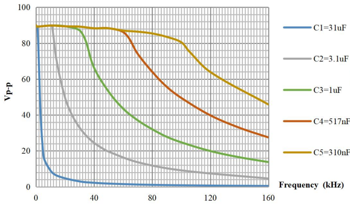
ATA-3040 容性负载曲线图
