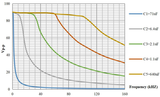
ATA-3090 容性负载曲线图
