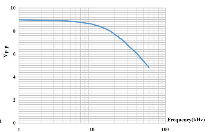
小信号幅频特性
