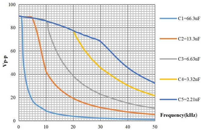
ATA-309B 容性负载曲线图
