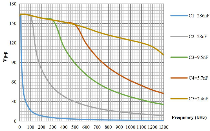
ATA-4011B 容性负载曲线图
