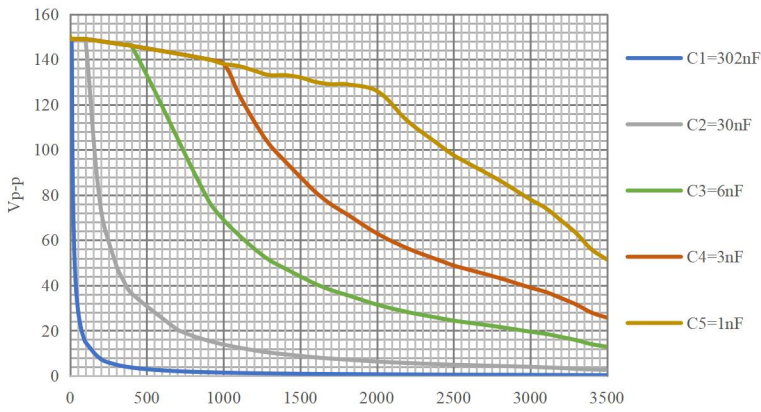
ATA-4315 容性负载曲线图
