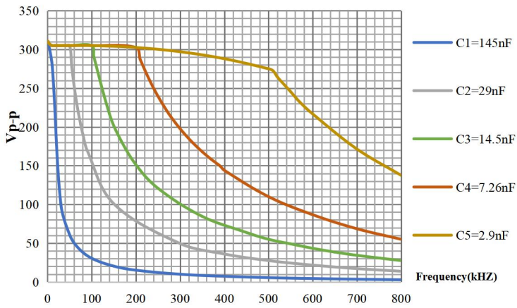
ATA-4051 容性负载曲线图
