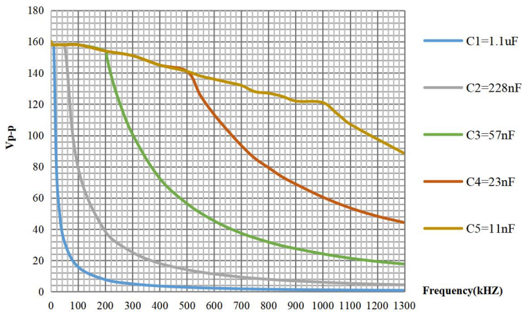
ATA-4014 容性负载曲线图
