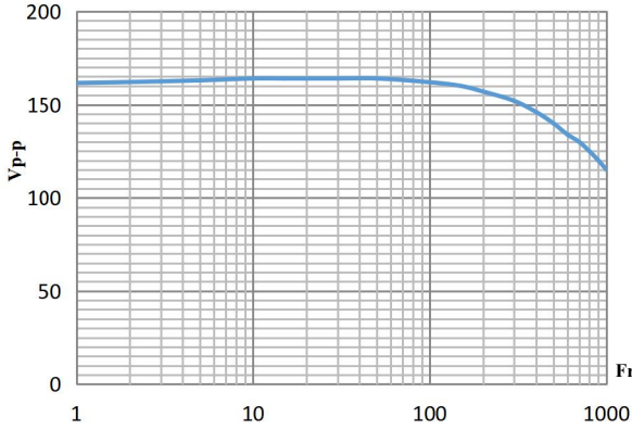
幅频特性 (最大输出电压 Vp-p)
