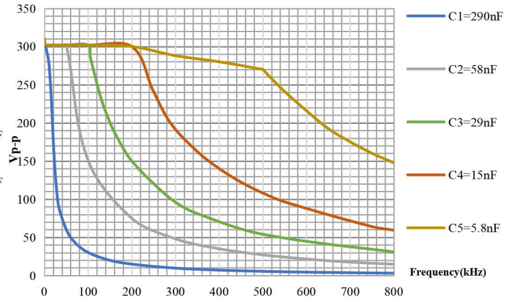
ATA-4052 容性负载曲线图
