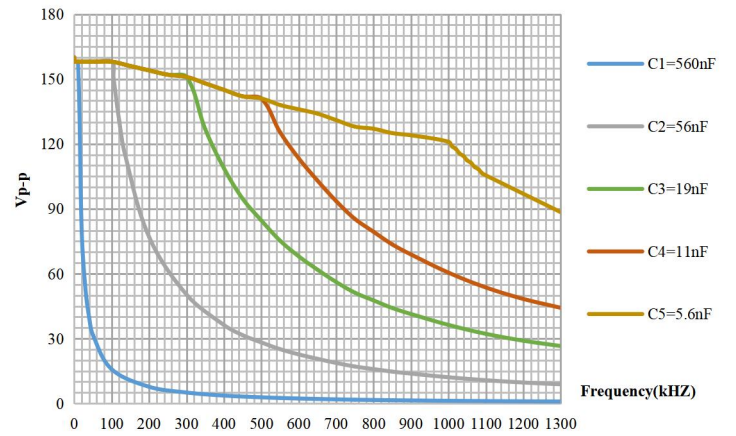
ATA-4012B 容性负载曲线图
